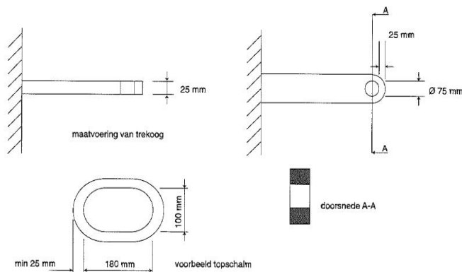
Figuur 32: maatvoering trekoog en topschalm
